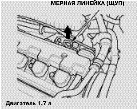
МЕРНАЯ ЛИНЕЙКА (ЩУП)
