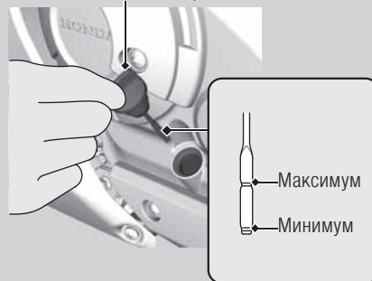
Крышка-щуп маслосливной горловины
